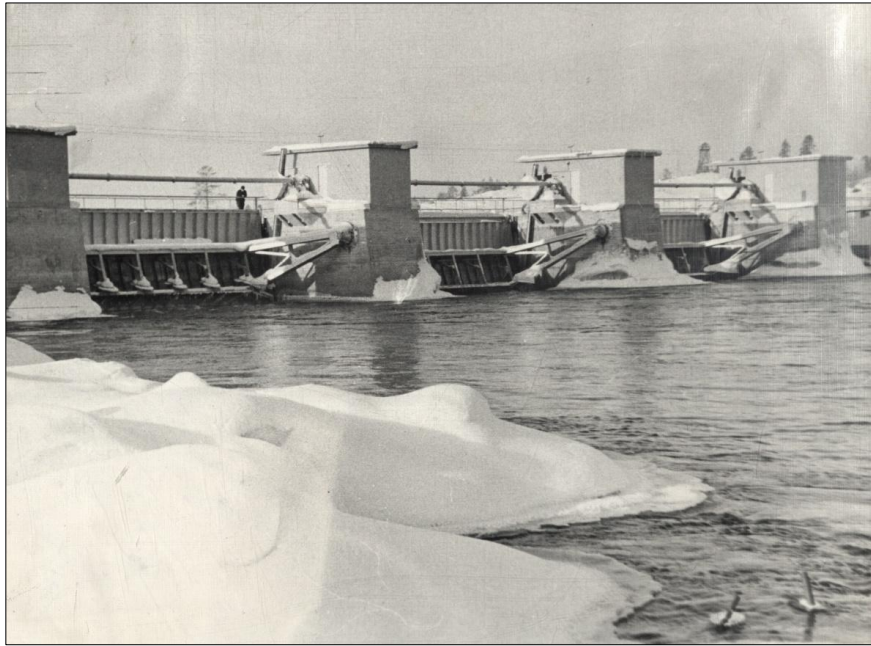
МОМ ОФ-15433/3529. ГЭС Янискоски. Регулирующее сооружение. 1956 г.
