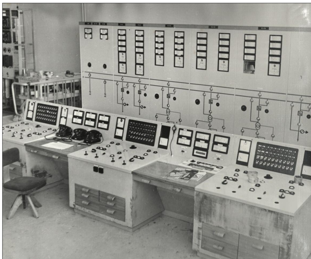
МОН ОФ-15433/3523. ГЭС Раякоски. Пульт управления. 1950-е гг.
